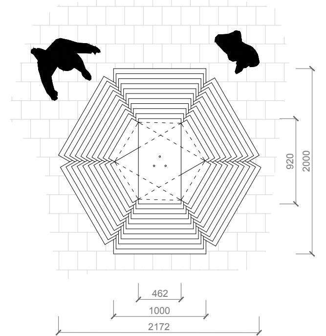
POHLAD HORNÝ m 1:50
