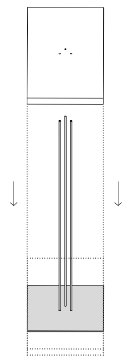
B. UKLADANIE PREDPRIPRAVENÝCH MATRACOV -uloženie na fixačnú výstuž
