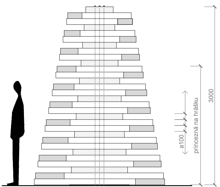
POHLAD BOČNÝ m 1:50
